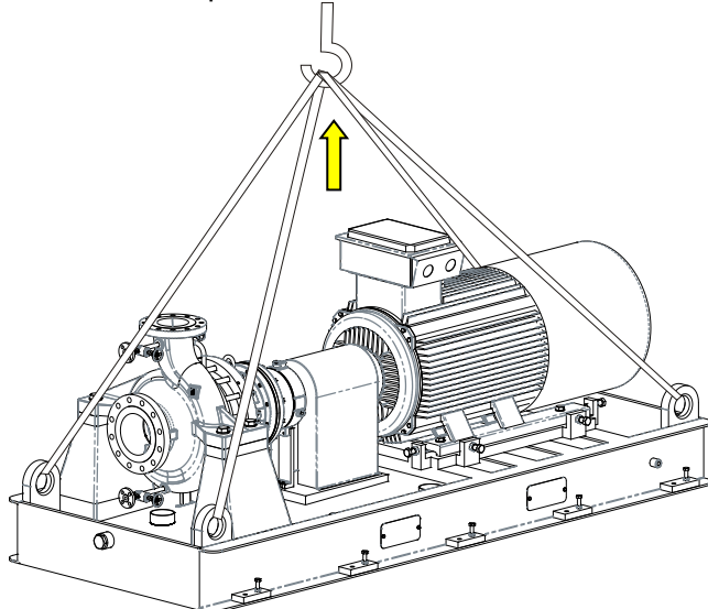
Pompa con basamento e motore
