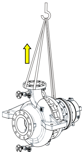
Pompa ad asse nudo
